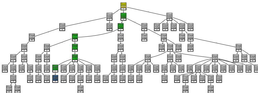
(b) graf przeszukiwań dla grafu z Rys. 2.6 wygenerowany przez algorytm A* używający odległości euklidesowej jako heurystyki
